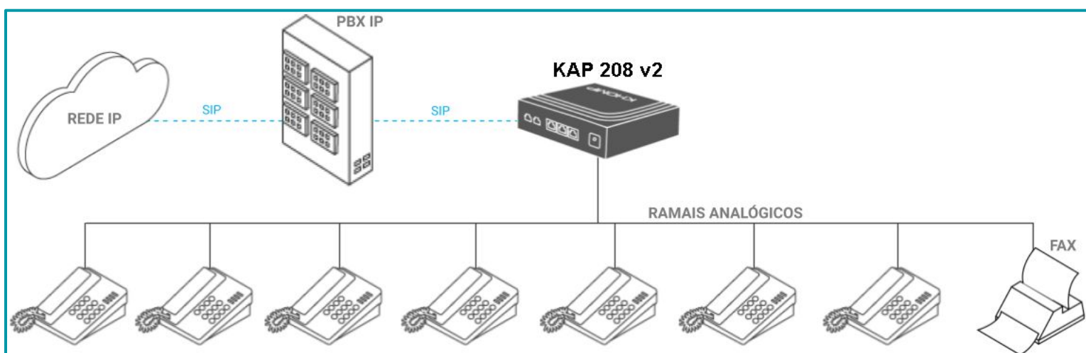
Legenda: Modelo de aplicação com PBX IP e múltiplas redes.
