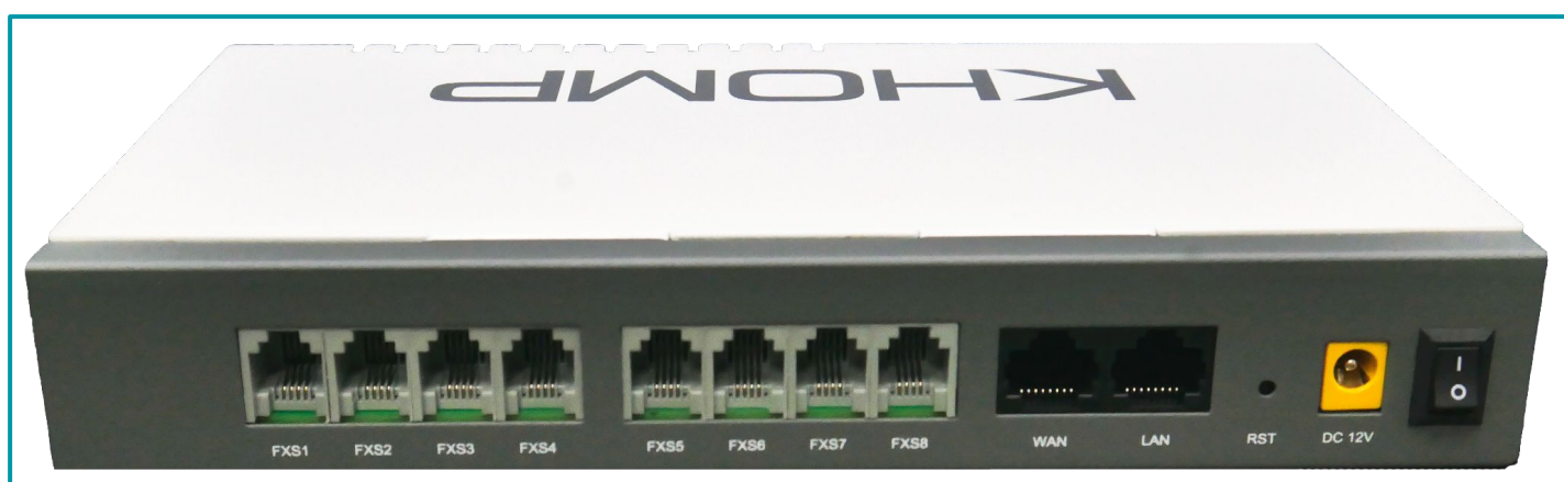
Legenda: Visão traseira com portas FXS, portas LAN e WAN, botão RTS, entrada para fonte de energia e botão interruptor para ligar ou desligar o produto.
